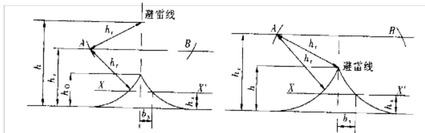
图B.0.1-2 单支避雷针的保护范围 ( h > hr )
