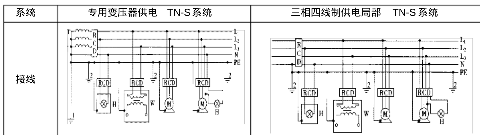
图 8.2.14 漏电保护器使用接线方法示意
