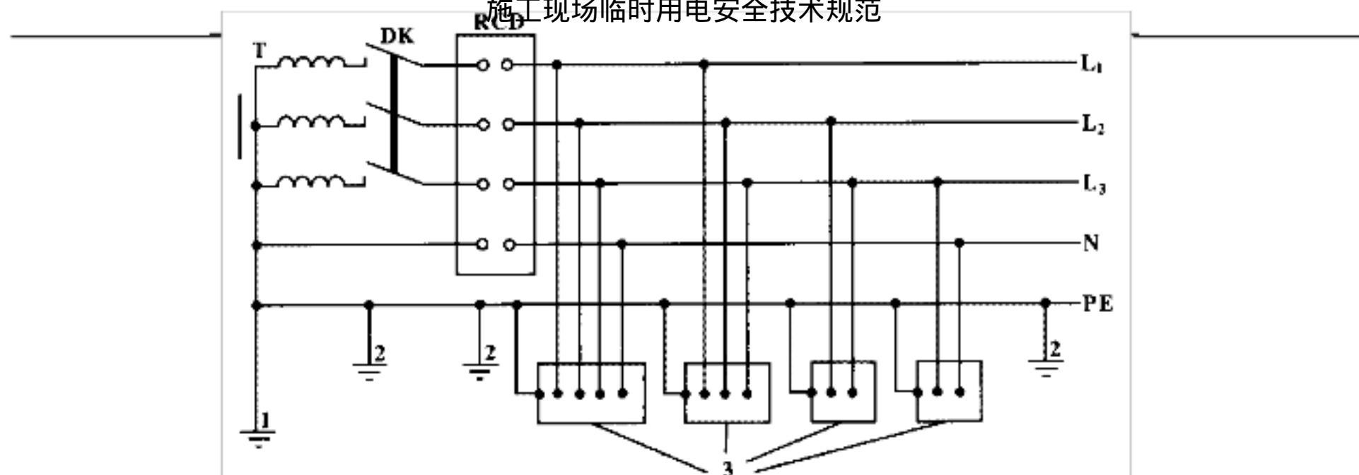
图5.1.1 专用变压器供电时 TN-S接零保护系统示意
